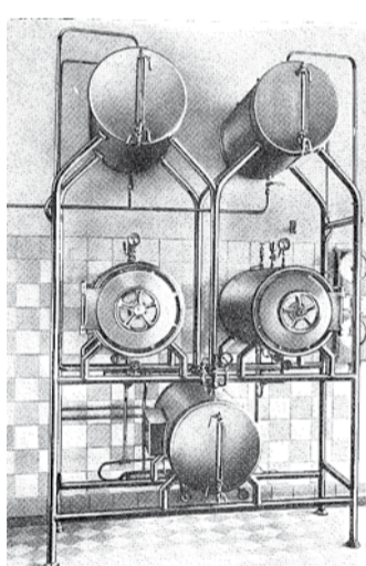
Un autoclave, v. 1900 Documentation du musée
